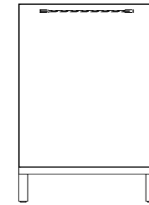
Waschbeckenschrank H517 L600 und Öffnungssystem Meuble lavabo H517 L600 et typologie d'ouverture
